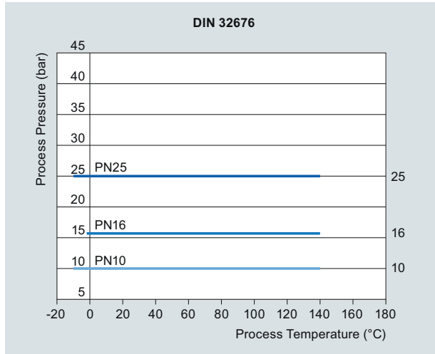
DIN 32676 flanges stainless steel (PN 10 ... PN 25)
