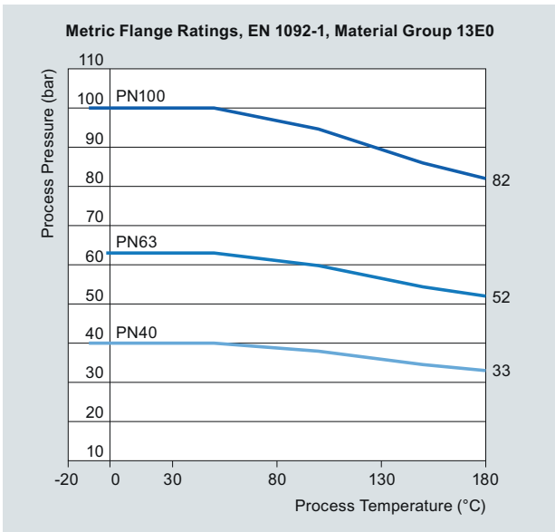
EN 1092 flanges stainless steel (PN 40 ... PN 100)
