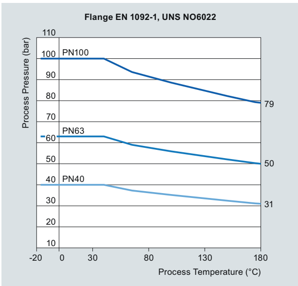
EN 1092 flanges Hastelloy C22 (PN 40 ... PN 100)
